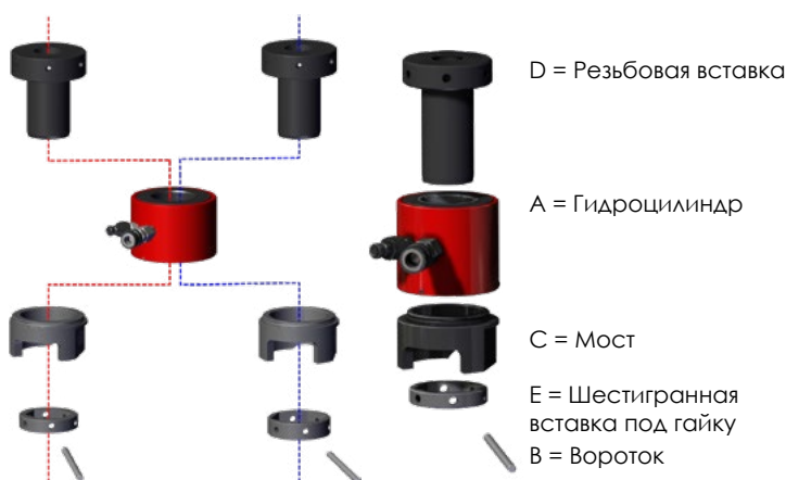
Принципиальная схема устройства шпильконатяжителя с пружинным возвратом серии SBT
